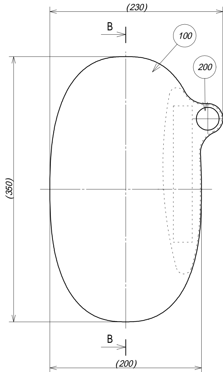
矢視 A
